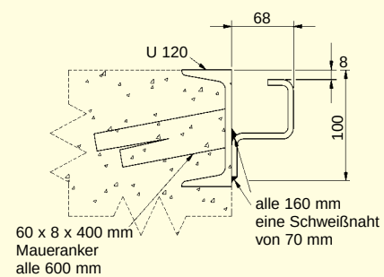
KBS-Führungsschiene
