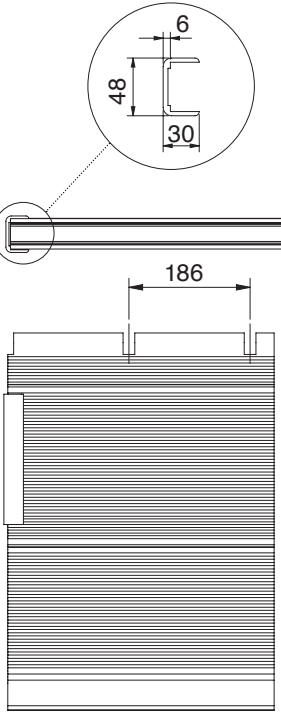
Randabschlussprofil RPB 40
