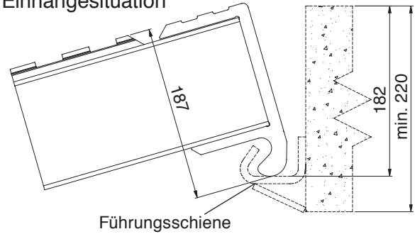
Auflager
