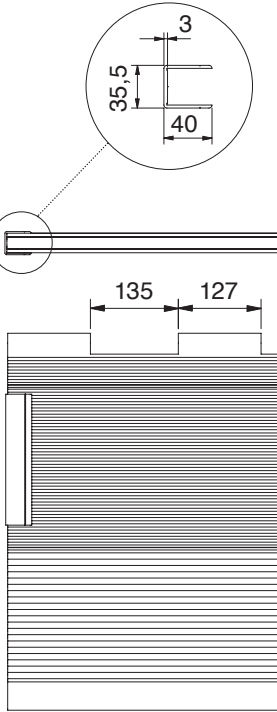
Randabschlussprofil RPB 30
