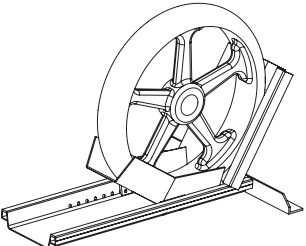
Gesichertes Rad
