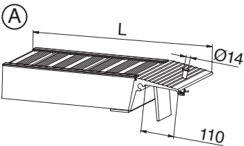
Auflagervariante
