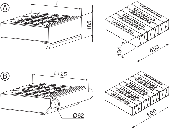
Auflagervarianten:
